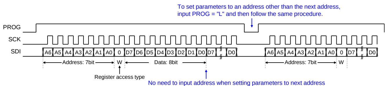
Fig. 4-40 OTP write parameter setting command
