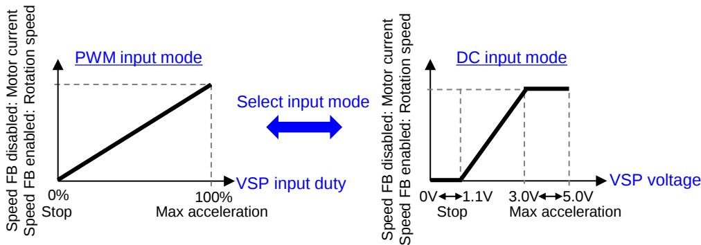
Fig. 4-10 PWM / DC input mode
